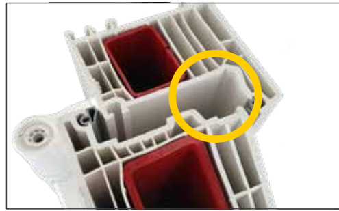
Wandungsstärke bis 3,5 mm für optimale Stabilität
